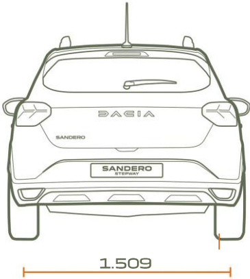
POGLED STRAGA
