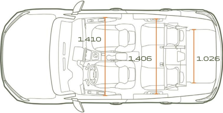
POGLED ODOZGO
