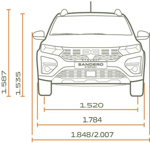
POGLED SPRIJEDA
