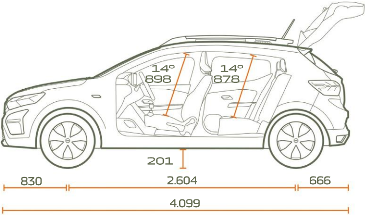
POGLED BOČNO
