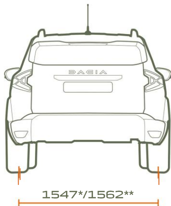
POGLED STRAGA
