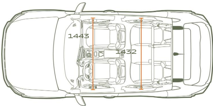
POGLED ODOZGO
