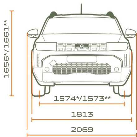
POGLED SPRIJEDA
