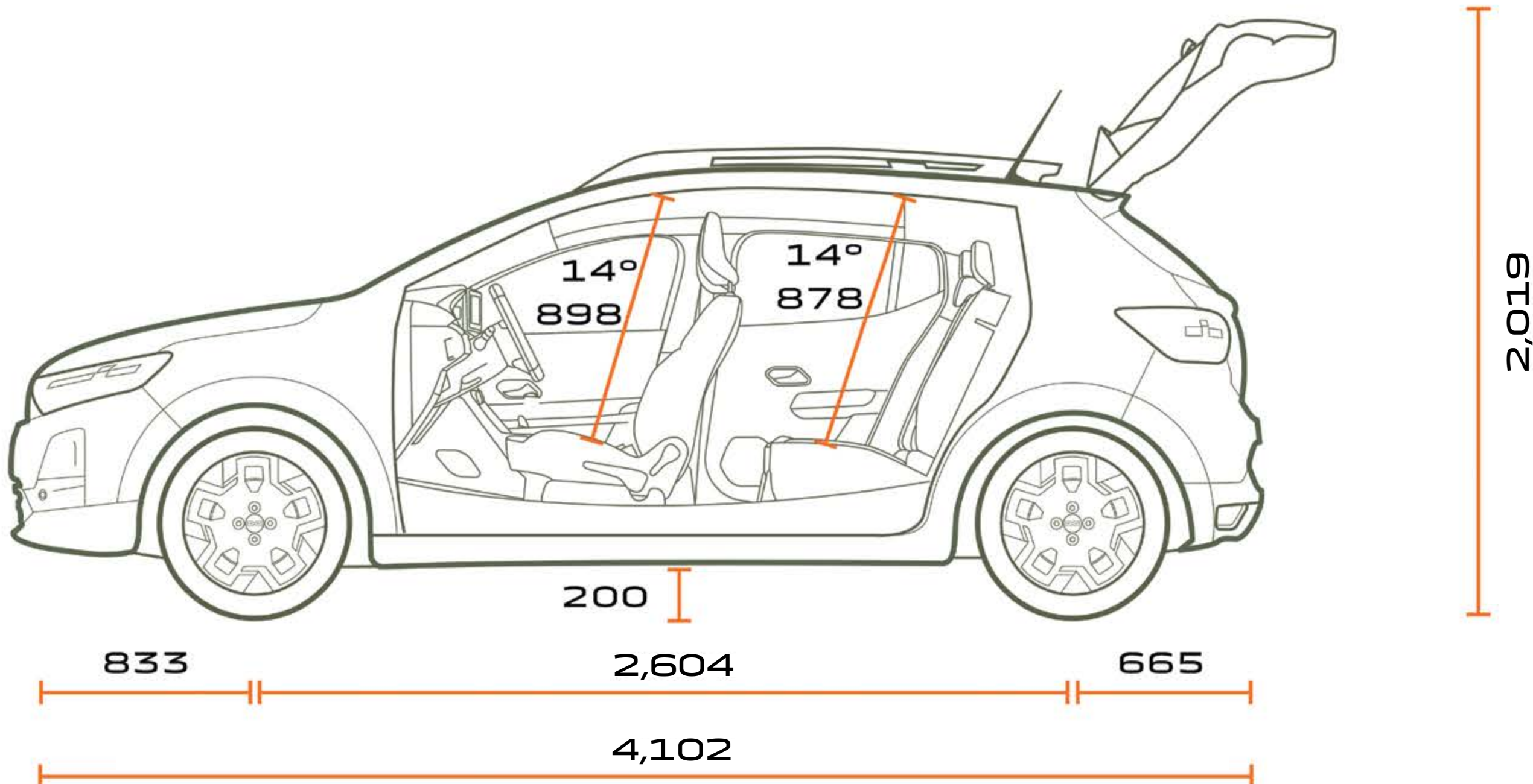
POGLED S BOČNE STRANE
