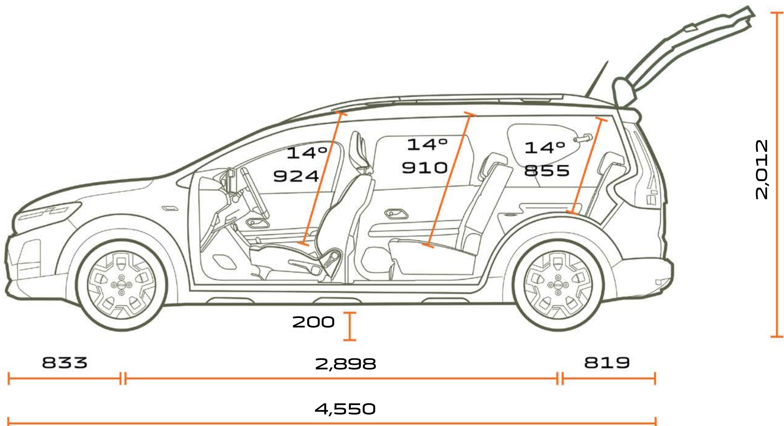
POGLED BOČNO NA IZVEDBU SA 7 SJEDALA
