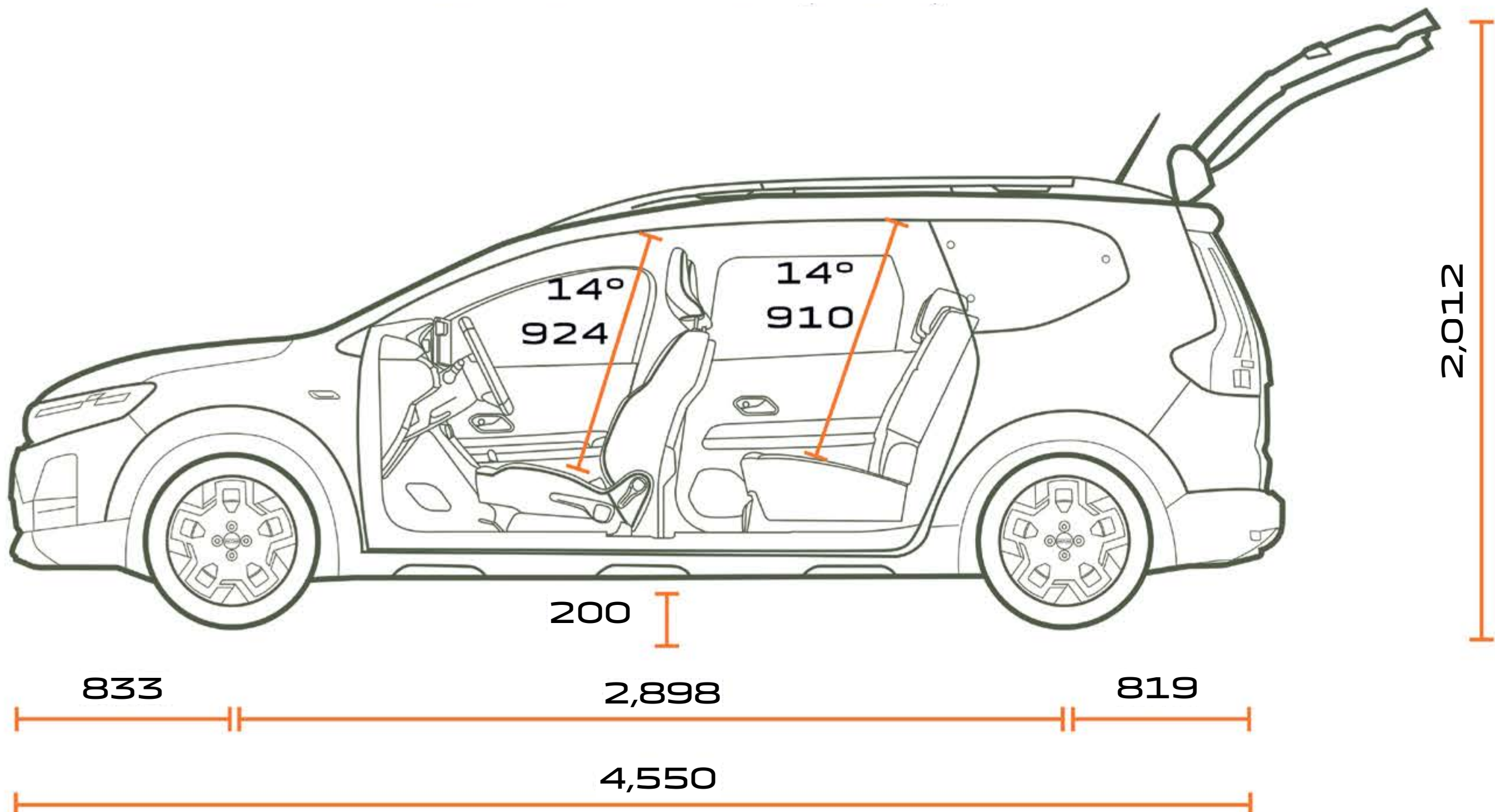
POGLED BOČNO NA IZVEDBU S 5 SJEDALA
