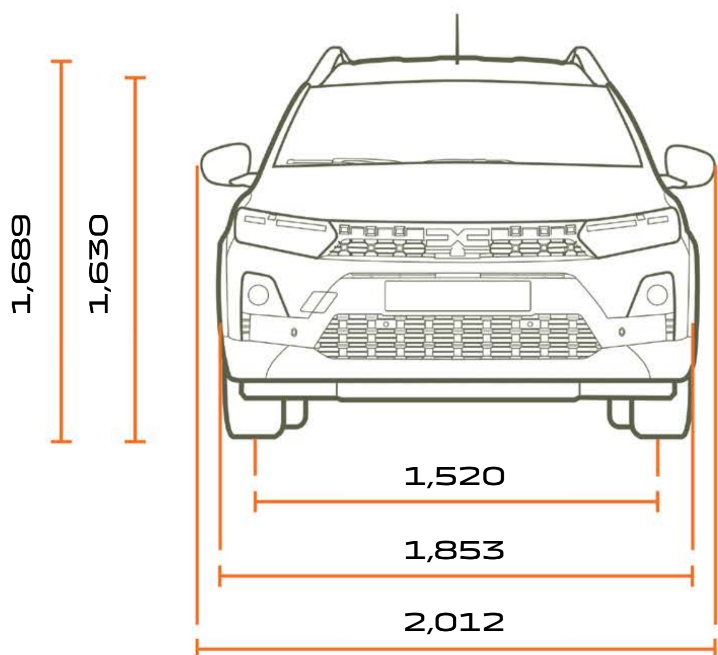
POGLED SPRIJEDA NA IZVEDBE S 5 I 7 SJEDALA
