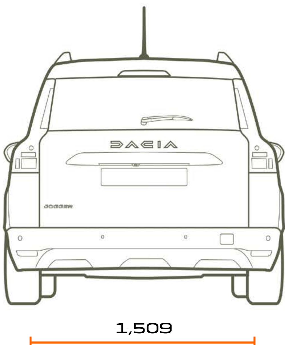
POGLED STRAGA NA IZVEDBE S 5 I 7 SJEDALA
