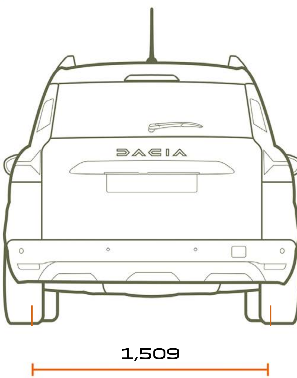
POGLED STRAGA NA IZVEDBE S 5 I 7 SJEDALA
