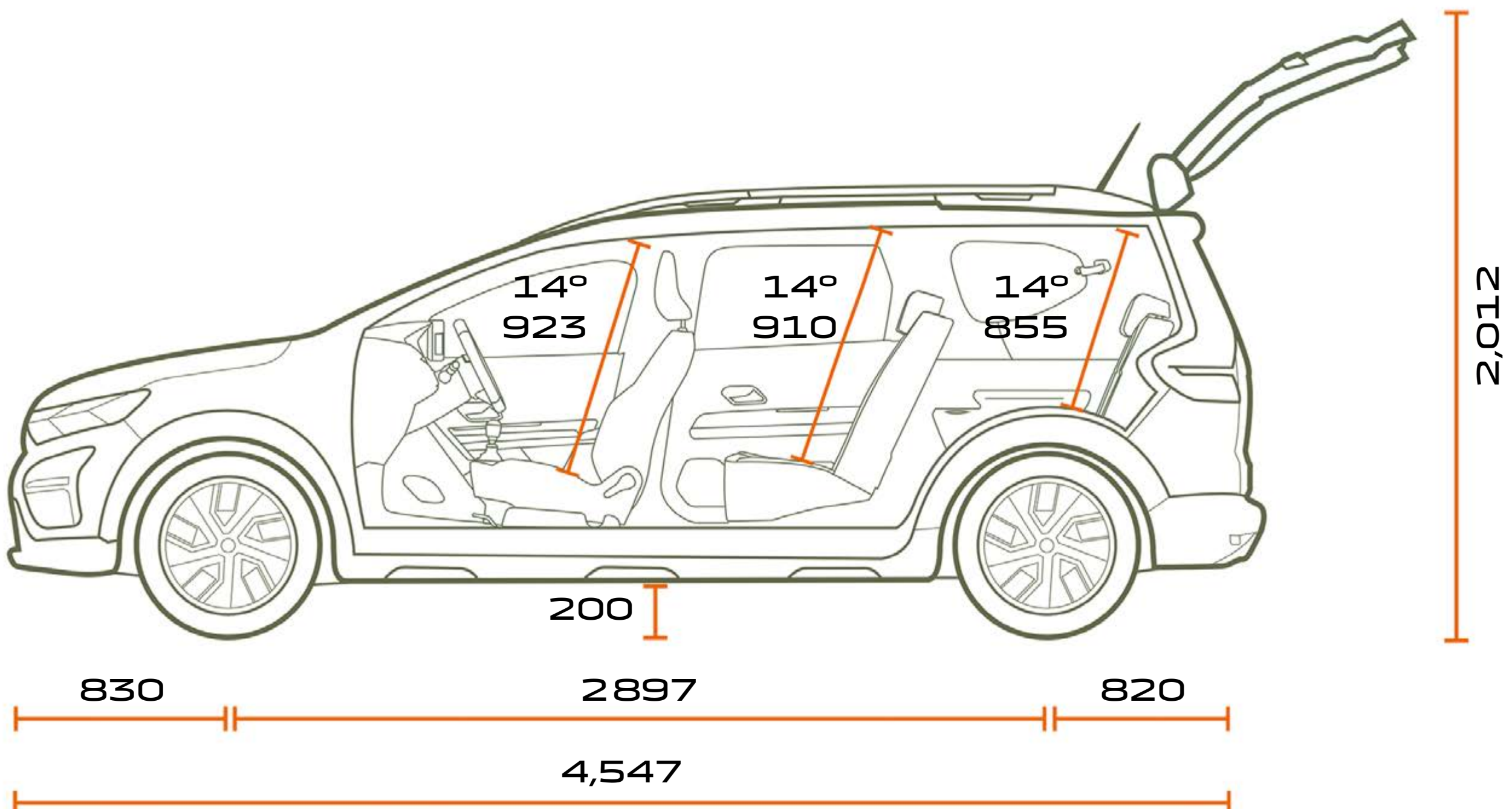
POGLED BOČNO NA IZVEDBU SA 7 SJEDALA
