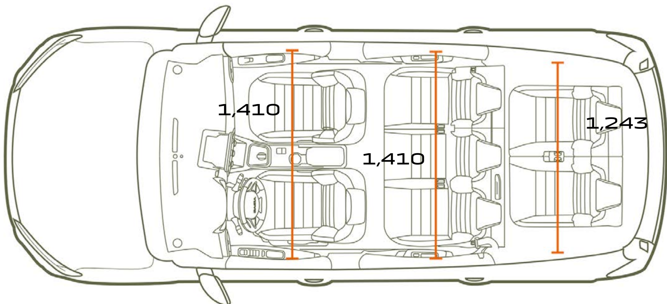
POGLED ODOZGO NA IZVEDBU SA 7 SJEDALA
