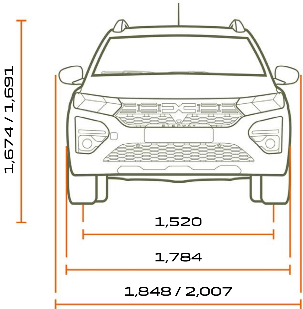
POGLED SPRIJEDA NA IZVEDBE S 5 I 7 SJEDALA
