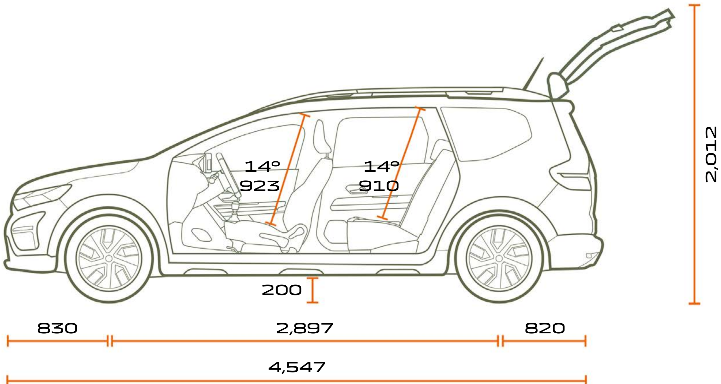
POGLED BOČNO NA IZVEDBU S 5 SJEDALA
